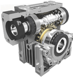
SONSUZ DİŞLİ REDÜKTÖRLER
